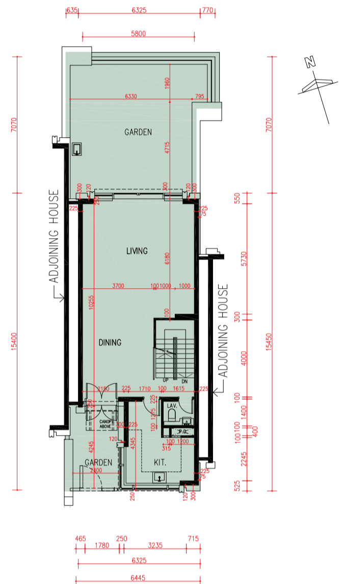
G/F Plan 地下平面圖
