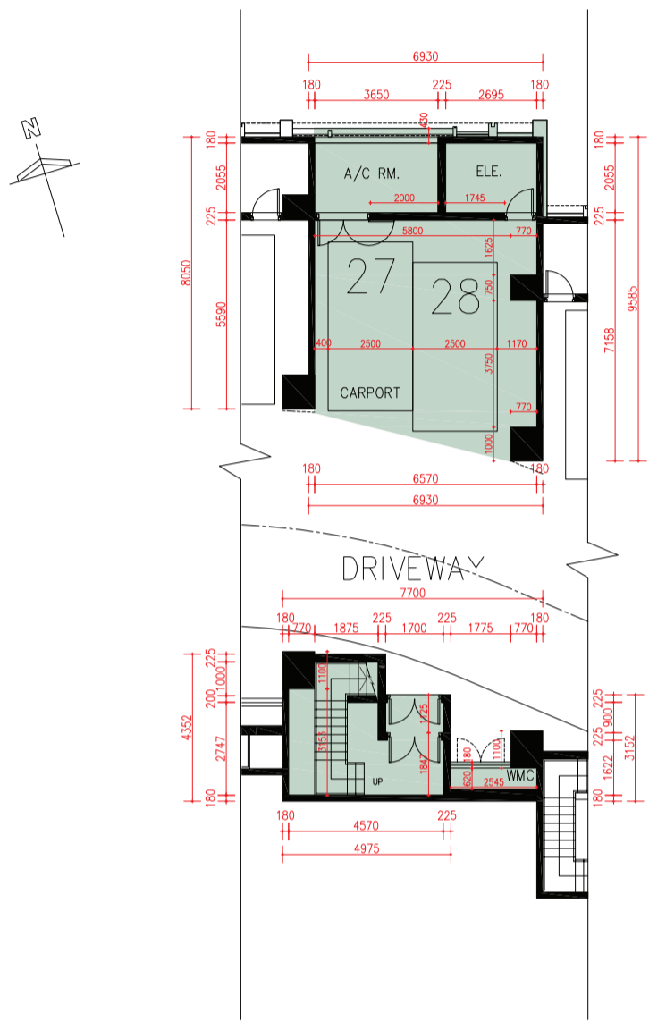
LG/F Plan 地下低層平面圖
