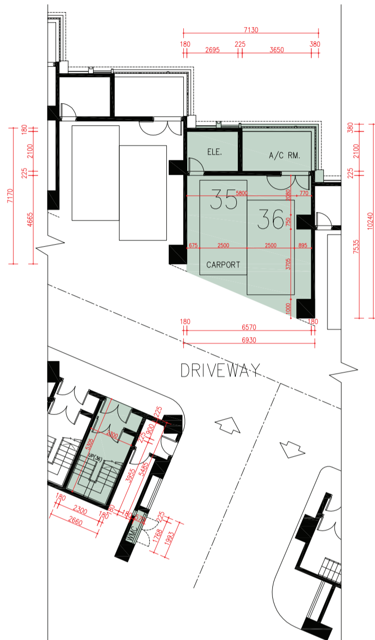
LG/F Plan 地下低層平面圖
